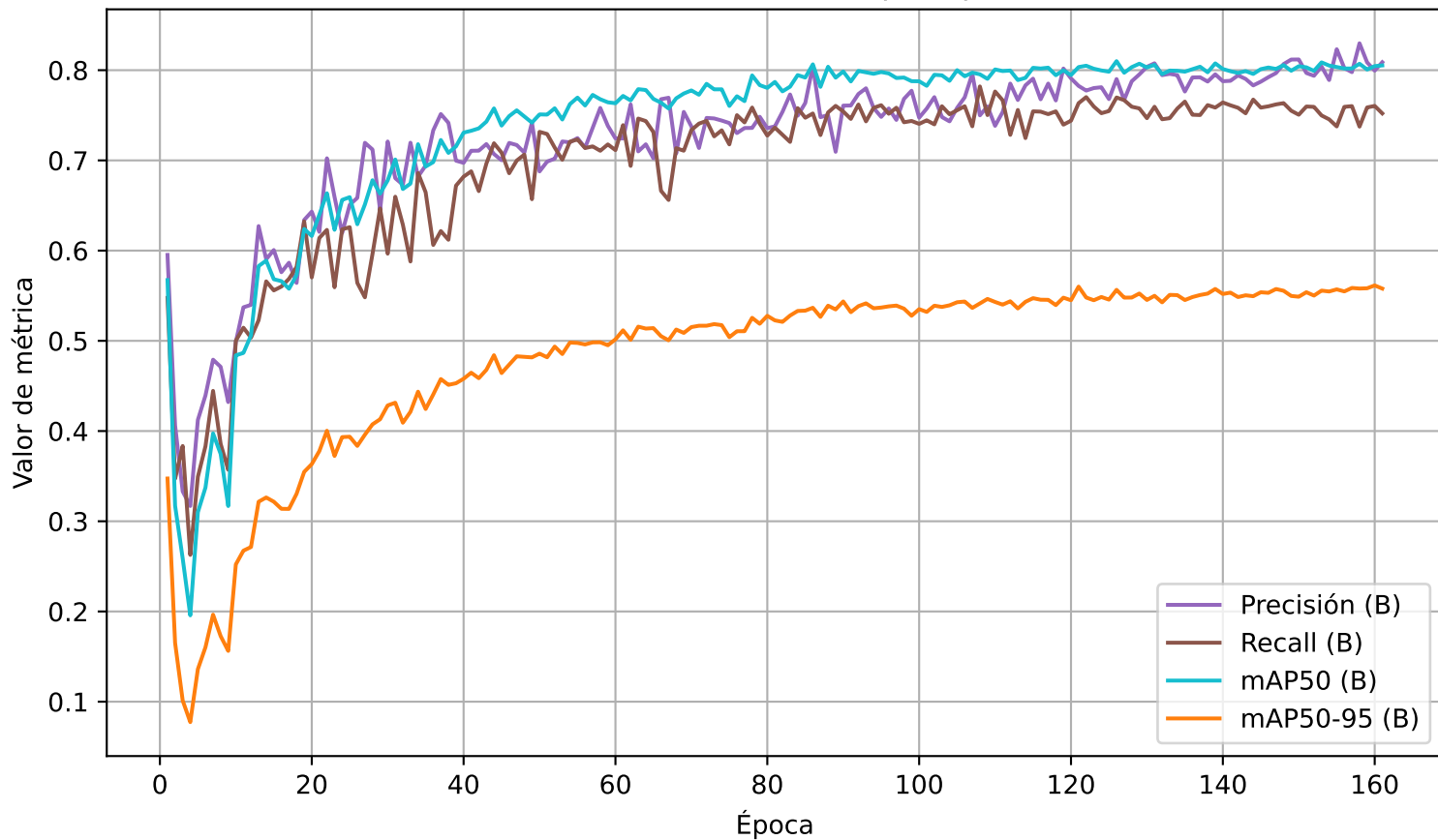
Métricas de evaluación por época
