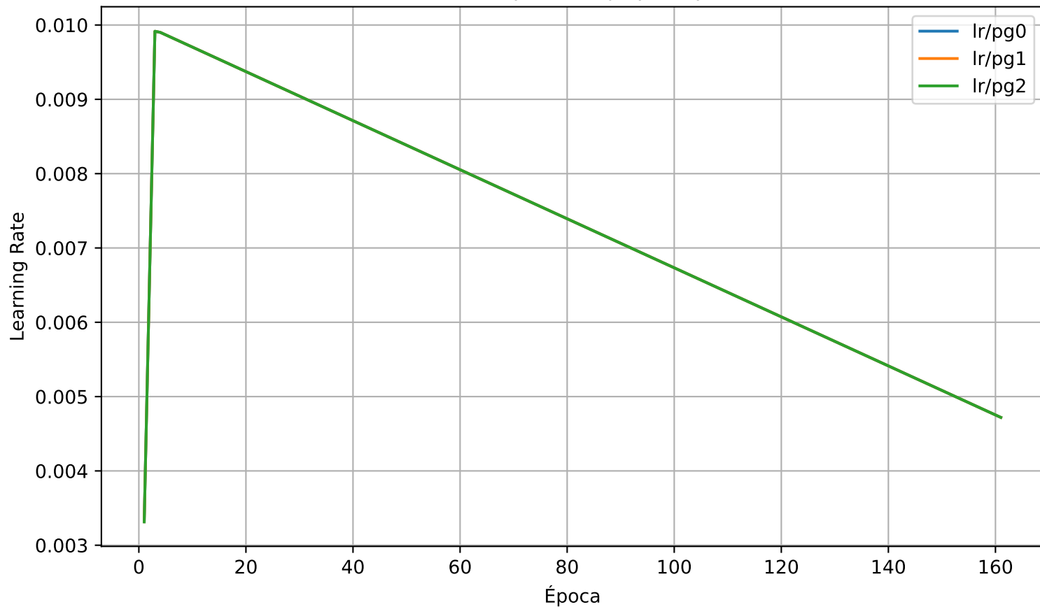
Tasas de aprendizaje por época
