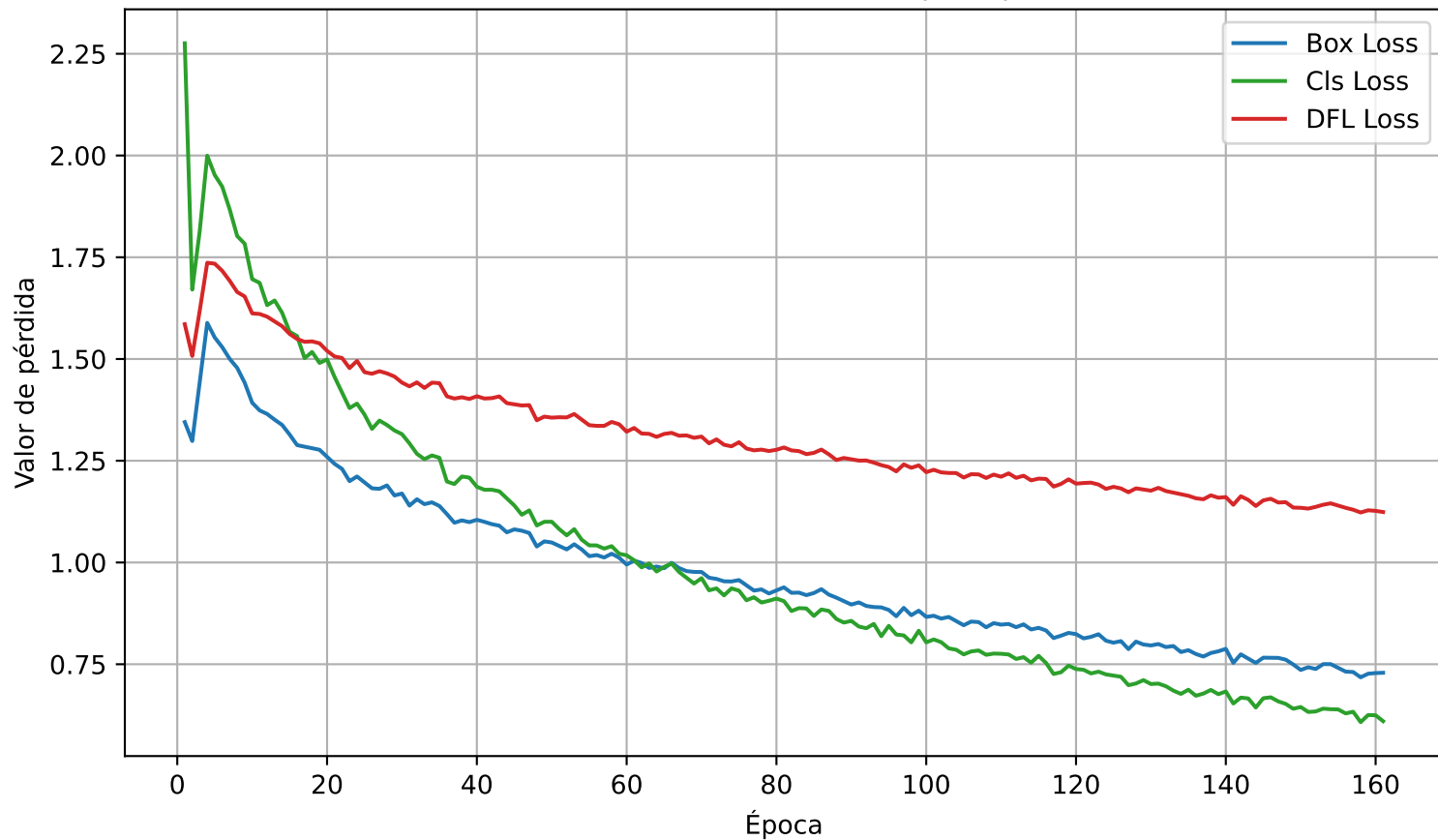
Pérdidas de entrenamiento por época
